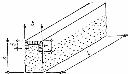
Rys. 5. Krawężnik drogowy rodzaju A
